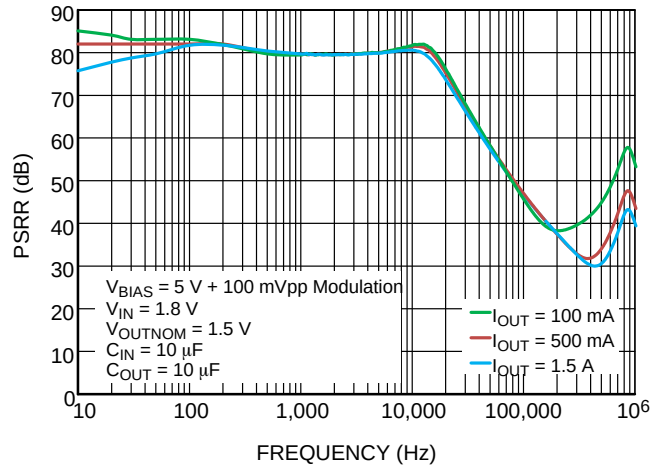
Figure 22. V_{BIAS} PSRR
