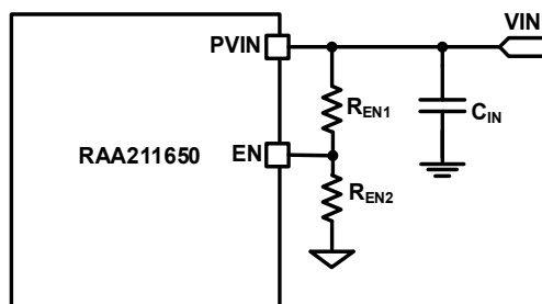
Figure 59. PVIN UVLO using EN
