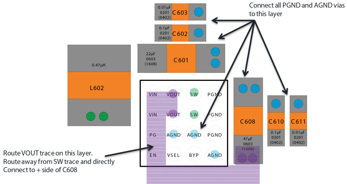
Figure 23. Layer 2
