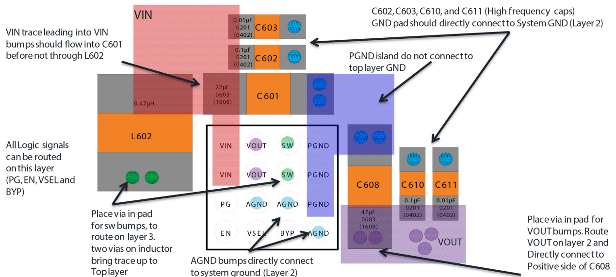
Figure 22. Top Layer
