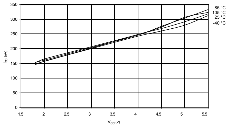
Figure 30-39. ADC Current vs. V CC (AREF = AV CC )
