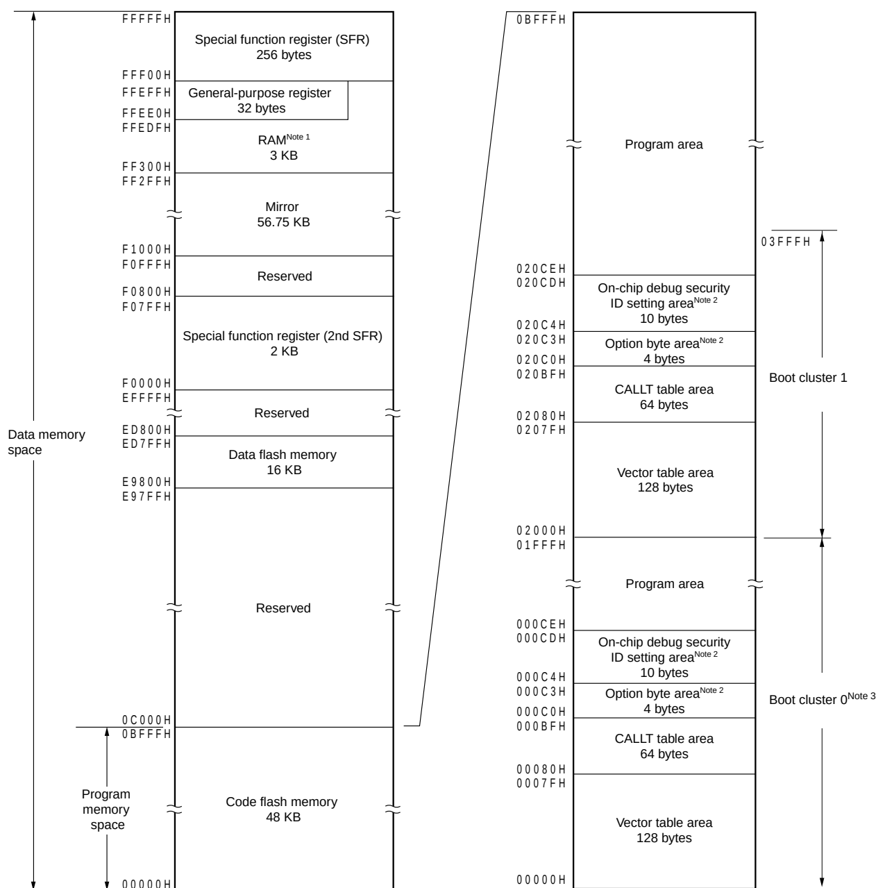
Figure 3-3. Memory Map (μPD78F1806, 78F1810, 78F1814, 78F1819)
