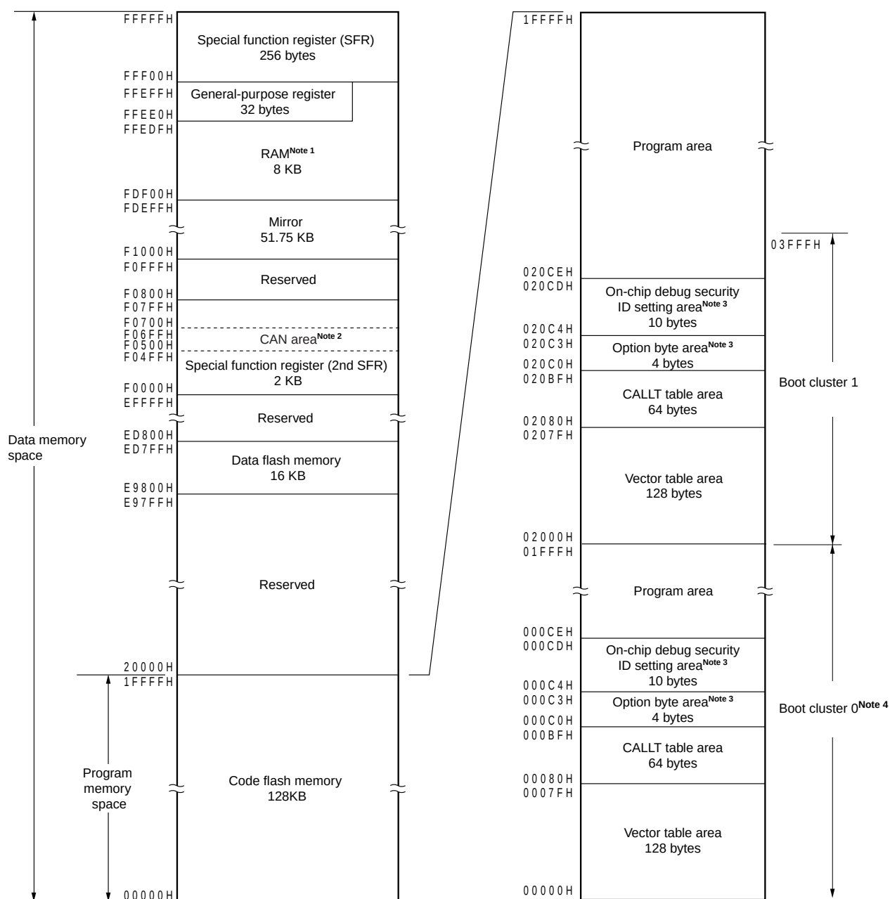
Figure 3-6. Memory Map ( \mu PD78F1817, 78F1822, 78F1825, 78F1828, 78F1833, 78F1838, 78F1843)
