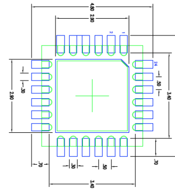
2.80 mm SQ EPAD
