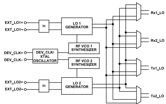
Figure 300. RF LO
