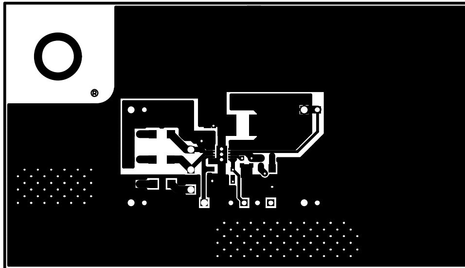
Figure 24. Top Layer
