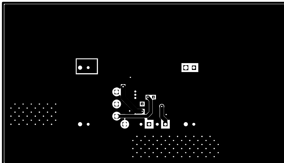
Figure 25. Bottom Layer
