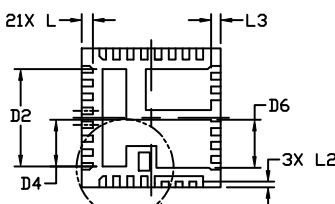
DETAIL B 2:1
