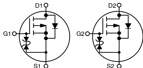
P-CHANNEL MOSFET
