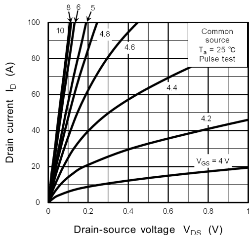
Fig. 9.1 I_D - V_{DS}
