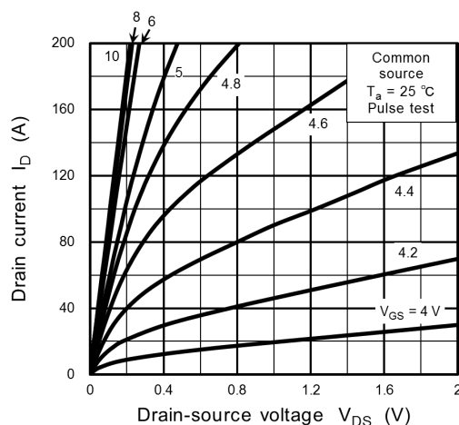
Fig. 9.2 I_D - V_{DS}
