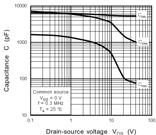
Fig. 9.8 Capacitance - V_{DS}
