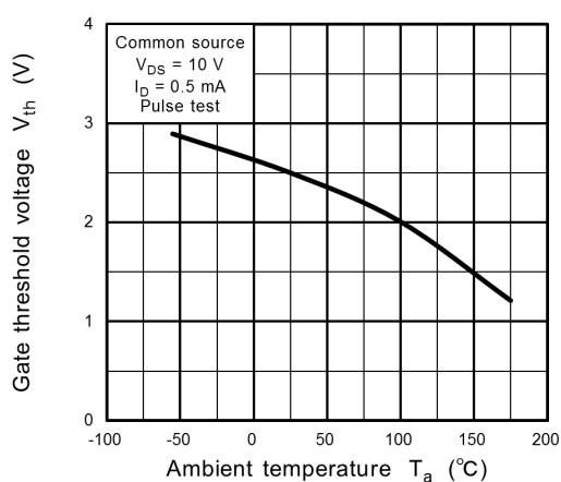
Fig. 9.9 V_{th} - T_a
