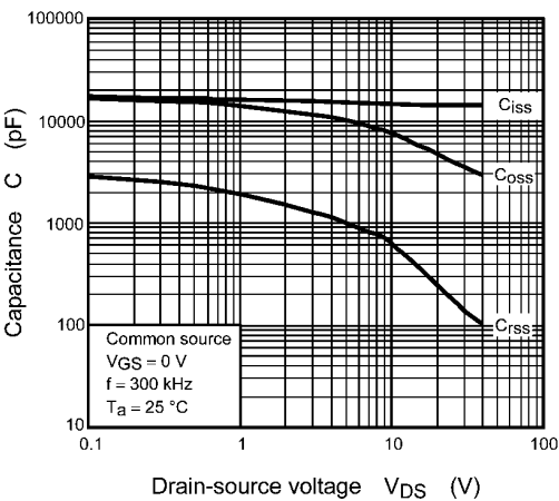
Fig. 9.8 Capacitance - V_{DS}
