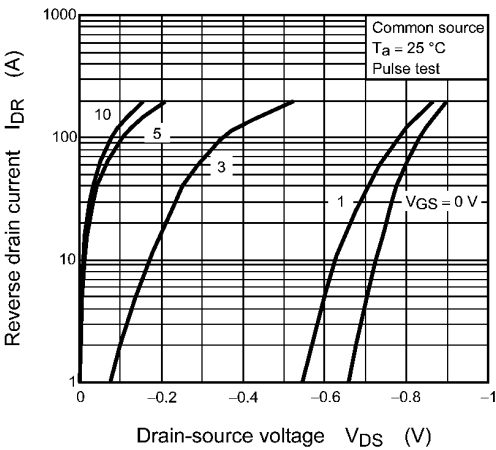
Fig. 9.7 I_{DR} - V_{DS}
