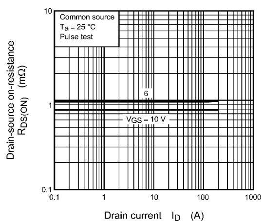
Fig. 9.5 R_{DS(ON)} - I_D
