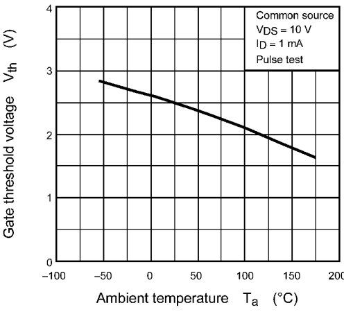
Fig. 9.9 V_{th} - T_a
