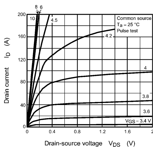
Fig. 9.2 I_D - V_{DS}
