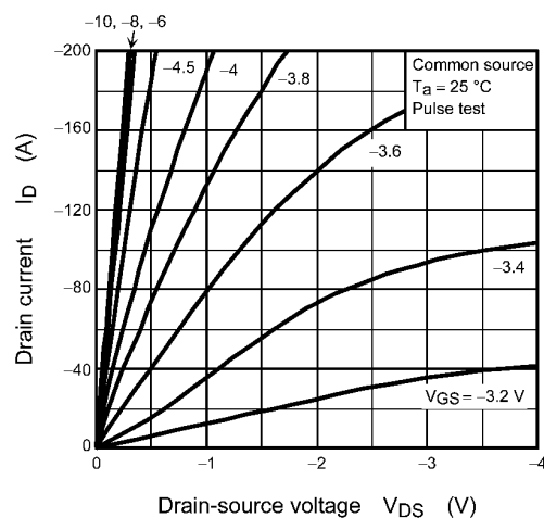
Fig. 9.2 I_D - V_{DS}
