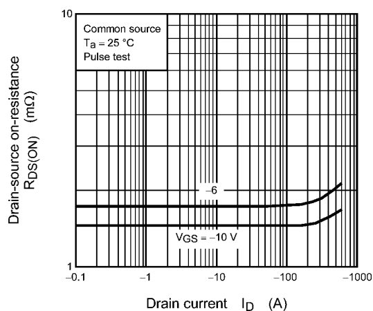
Fig. 9.5 R_{DS(ON)} - I_D
