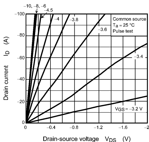
Fig. 9.1 I_D - V_{DS}
