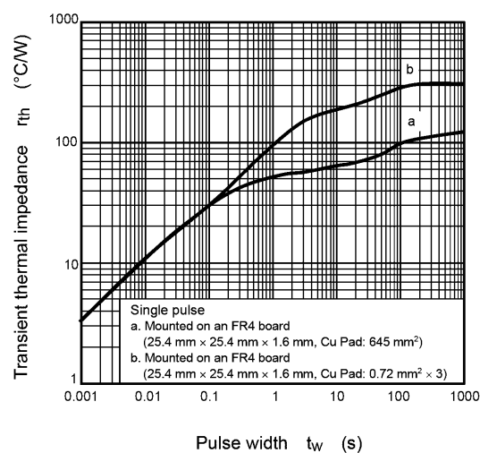
Fig. 8.13 r_{th} - t_w
