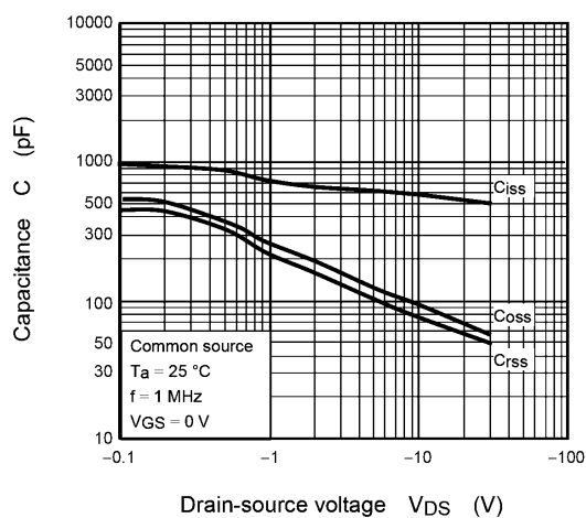
Fig. 8.10 C - V_{DS}
