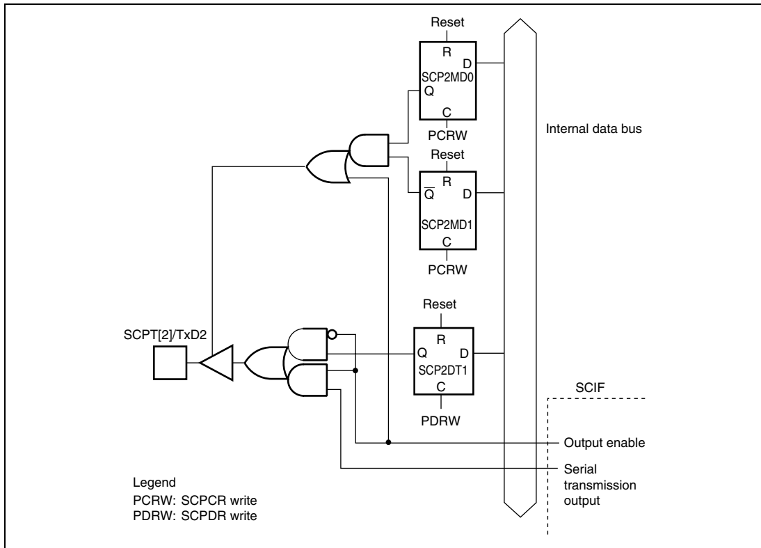
Figure 16.3 SCPT[2]/TxD2 Pin
