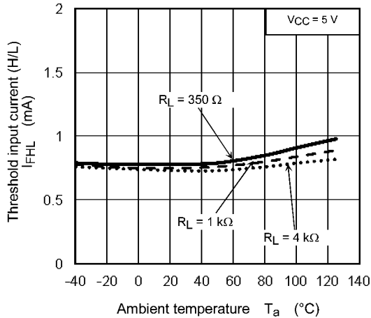
Fig. 12.2.7 I_{FHL} - T_a
