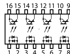
PS2806-4
