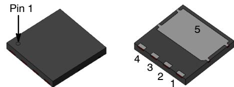
PQFN4 8X8, 2P (Power88) CASE 483AP
