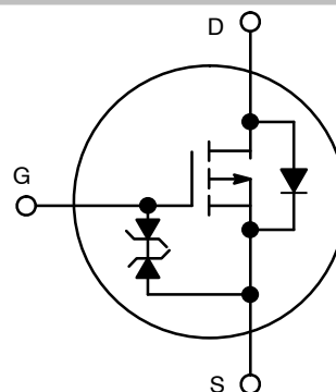
P-Channel MOSFET
