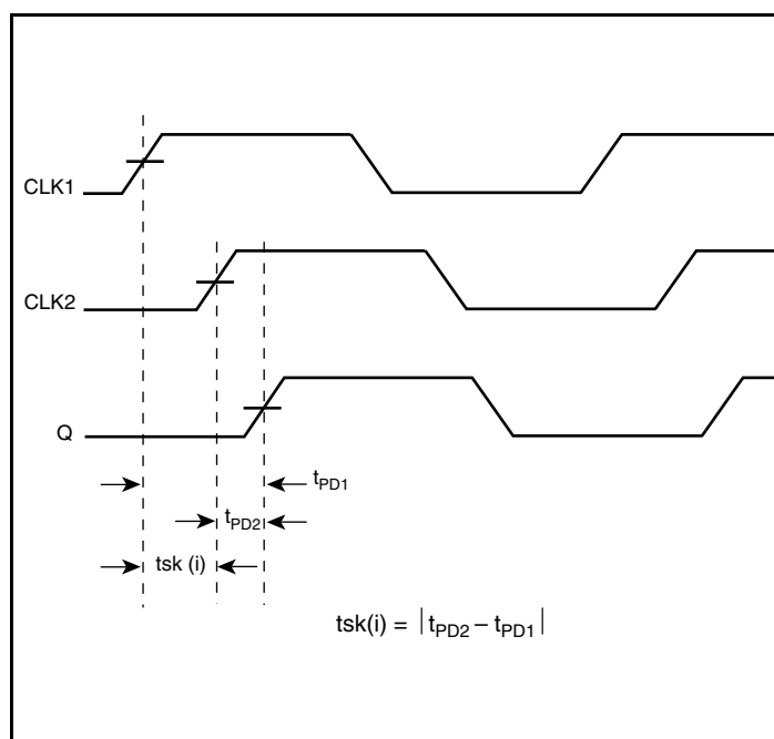
Input Skew
