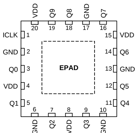
20-pin VFQFPN
