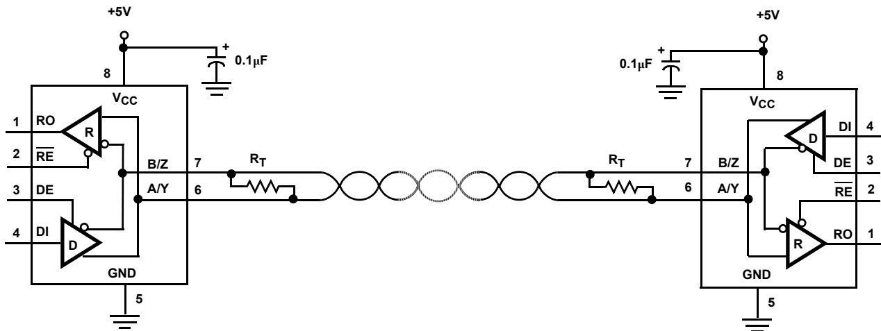
ISL8483E, ISL8485E
