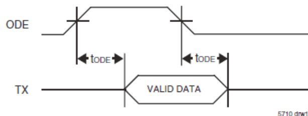
Figure 11. Output Driver Enable (ODE)
