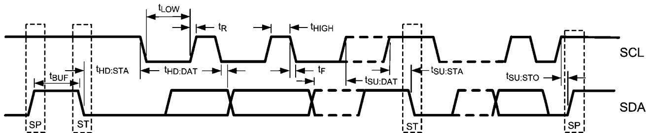
SMBus Timing Parameters
